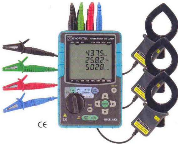
MEDIDOR DE POTENCIA TRIFASICO MOD. 6300 MIDE VOLTAJE, CORRIENTE, POTENCIA ACTIVA, REACTIVA Y APARENTE, ENERGIA ACTIVA, APARENTE, REACTIVA, FRECUENCIA, MEDICION DE DEMANDA., COMUNICACIÓN A PC, CAT III 600 V.
